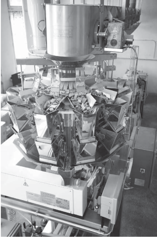
Die kompakte Verpackungslösung für die Hundekekse mit der Mehrkopfwage CCW-SE von Ishida.
