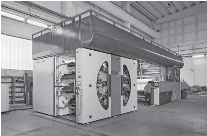
Die EVO XD-Baureihe von KBA-Flexotecnica adressiert mit vielen Innovationen die heutigen Marktanforderungen im Flexodruck.
