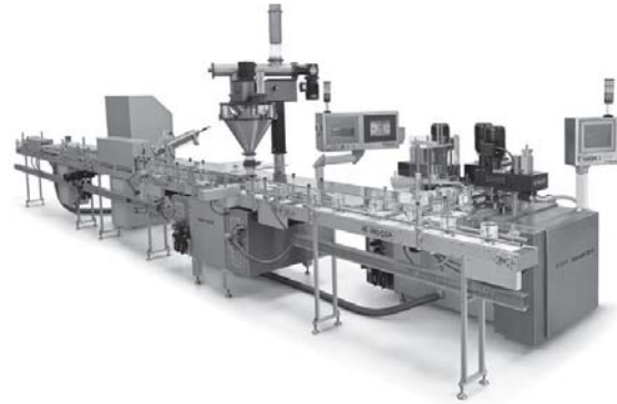
Indosa Milchpulveranlage.
