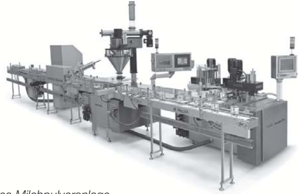
Indosa Milchpulveranlage.
